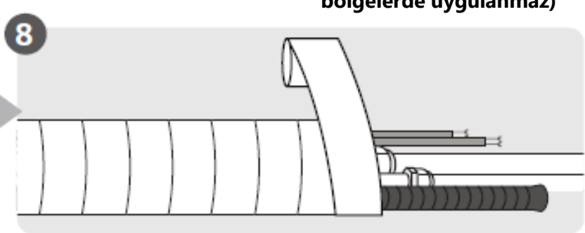
8 Boru Tesisatını ve Kabloyu Sarın (Kuzey Amerika'da bazı bölgelerde uygulanmaz)
