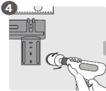
4 Duvara Delik Açın
