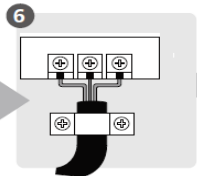
6 Kablo Bağlantısını Bağlayın (Kuzey Amerika'da bazı bölgelerde uygulanmaz)
