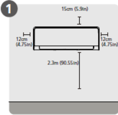
1 Kurulum Yerini Seçin
